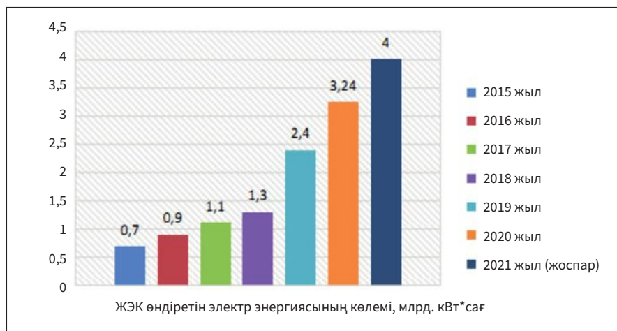
4-сурет. ҚР-да 2015-2021 жж. ЖЭК электр энергиясын өндіру серпіні
