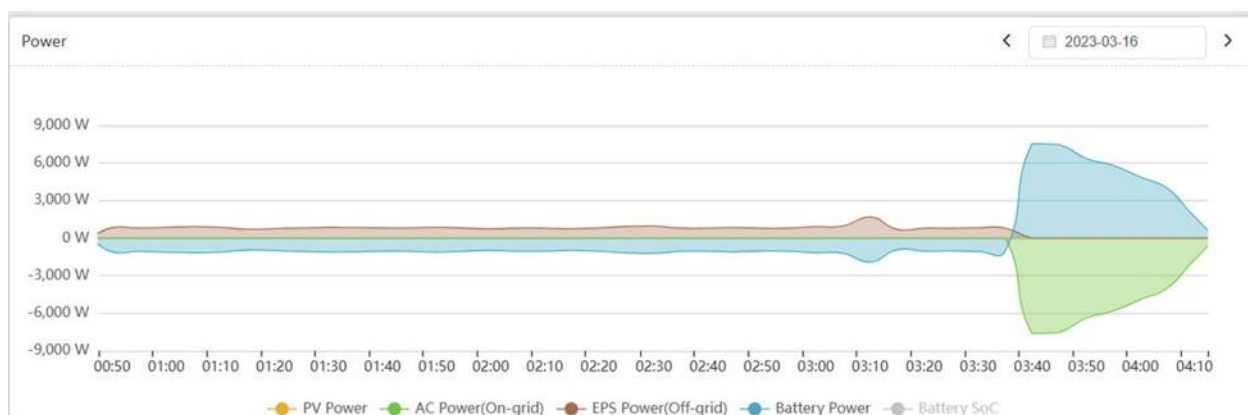
Алматыдағы гибриді ФЭС-те 16.03 уақыт аралығы
